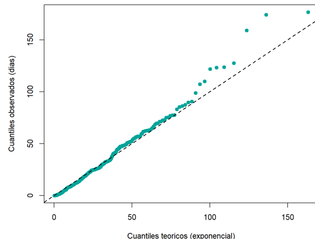
Figura 7. QQ exponencial de los tiempos entre eventos para M \geq 7,0 .
